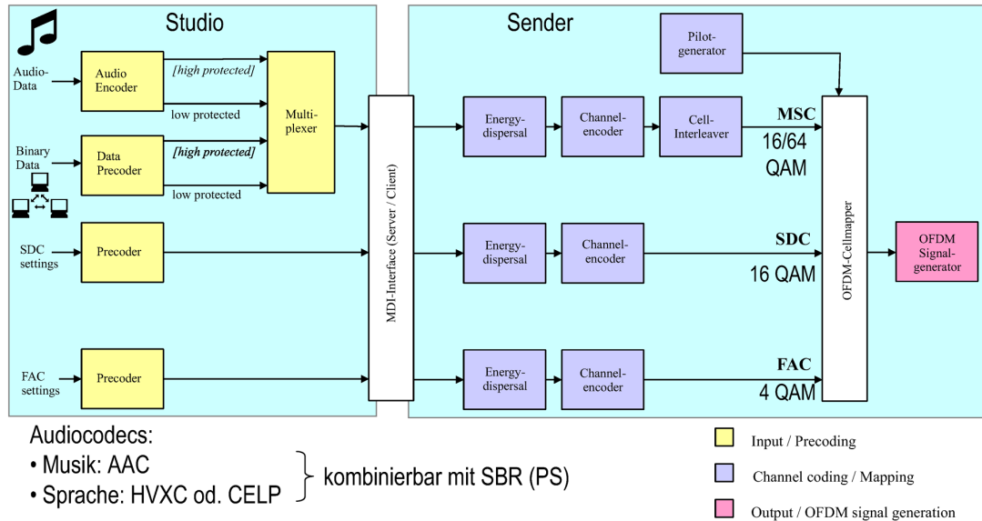
Abbildung 4.7: Aufbau eines DRM+-Signalgenerators
